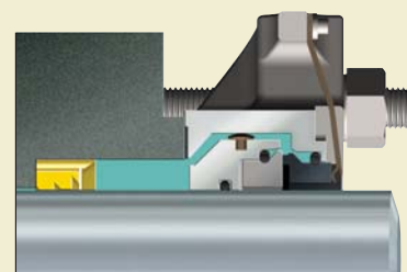
442 Delad tätning med SpiralTrac™
