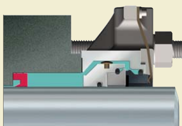
442 Delad tätning med 14K
