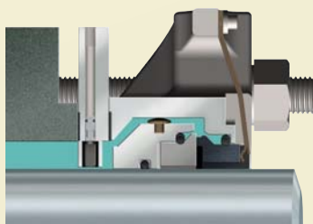
442 Delad tätning med ISS skyddstätning
